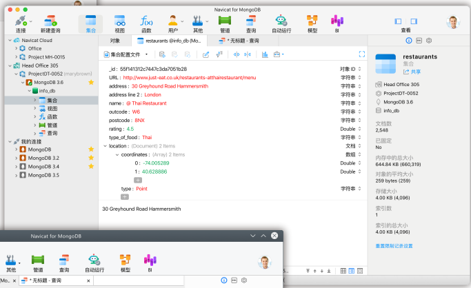
macOS 版本
