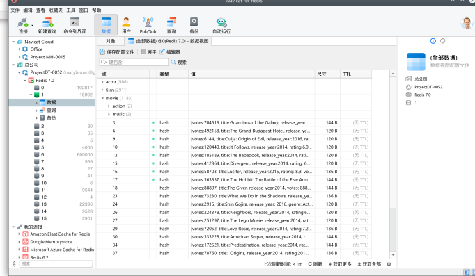
Linux 版本
